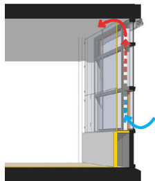
klimaatgevel winter
